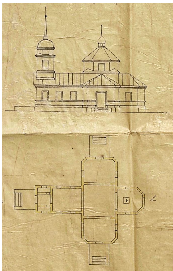
Проект деревянной церкви в с. Сторожевое. 1892 г. ГАКО
