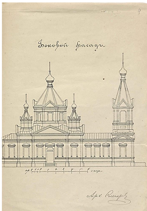
Проект Михаилоархангельского храма с. Быканово (боковой фасад).
