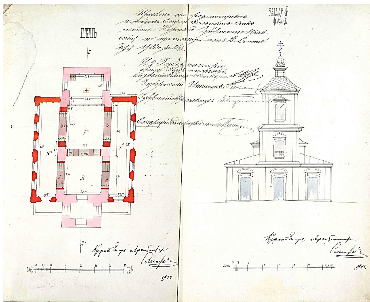
Проект западного фасада (справа) и архитектурно-строительный чертеж (слева) Казанской церкви с. Переверзевка. 1903 г. ГАКО
