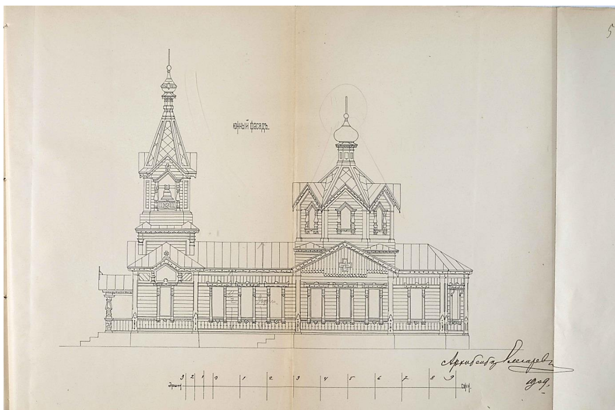
Проект деревянной церкви в д. Маховой Колодезь (южный фасад). 1909 г. ГАКО
