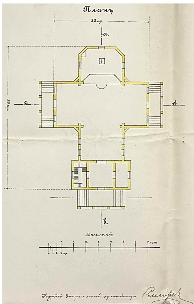
Проект Успенской церкви с. Кулига. Вид сверху. 1899 г. ГАКО
