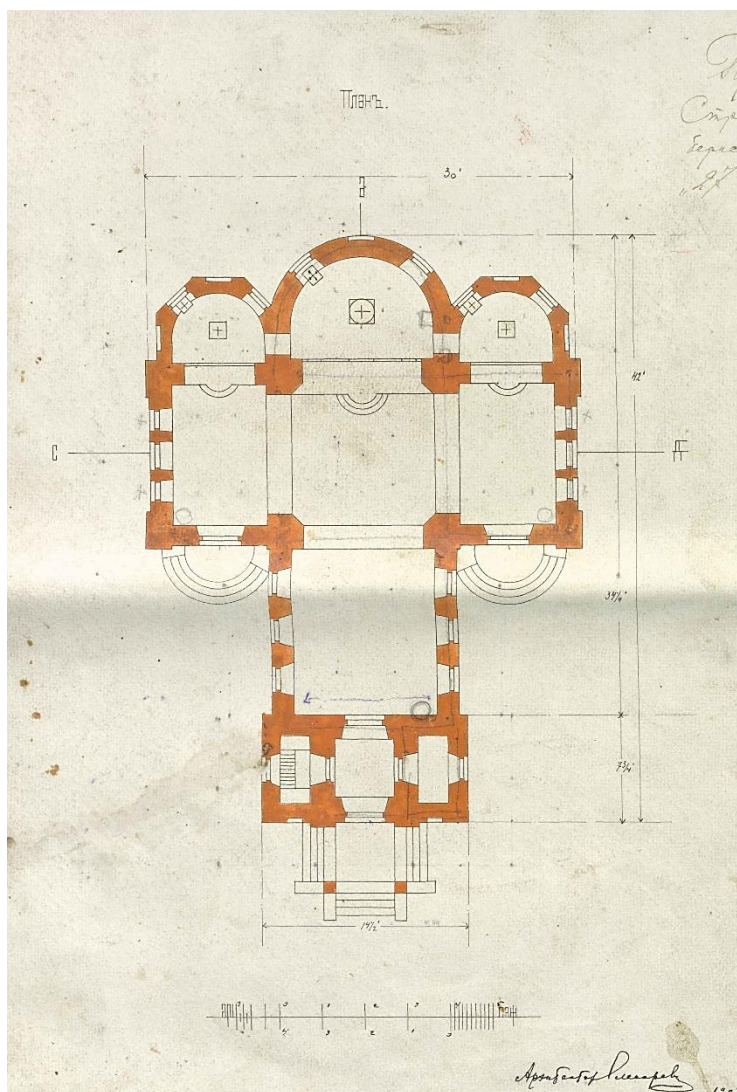
План каменного Христорождественского храма с. Камышное. 1907 г. Автор В. Г. Слесарев. ГАКО
