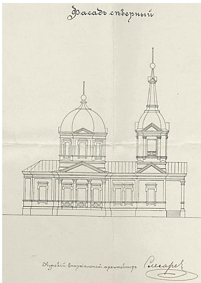
Проект Успенской церкви с. Кулига. 1899 г. ГАКО
